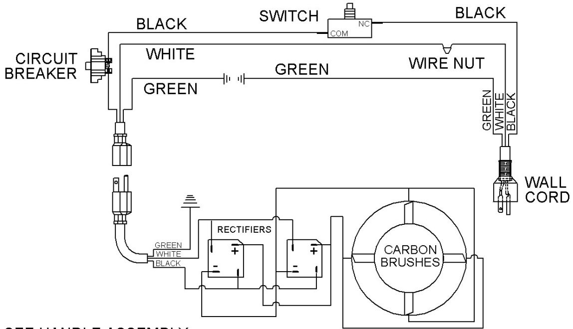
WIRE DIAGRAM - 120 VOLT
