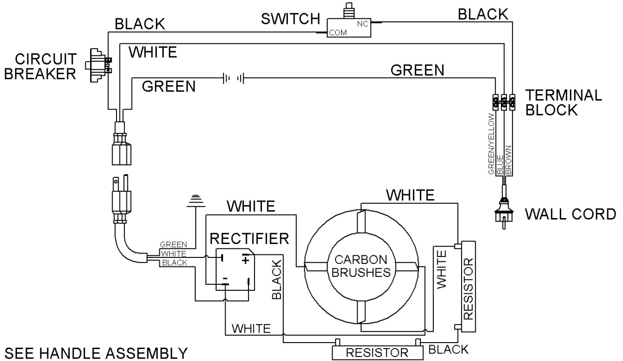
WIRE DIAGRAM - 240 VOLT
