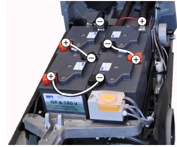
Schéma de montage pour 4 batteries
