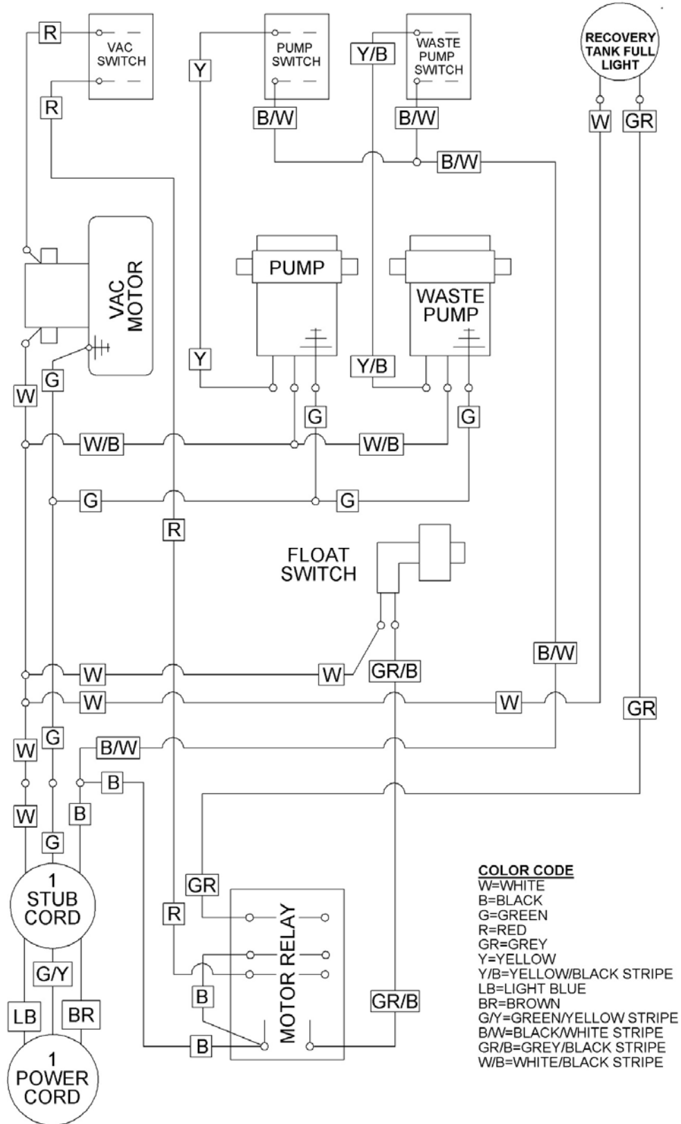
RALLY 1200 240 VOLT WIRING DIAGRAM
