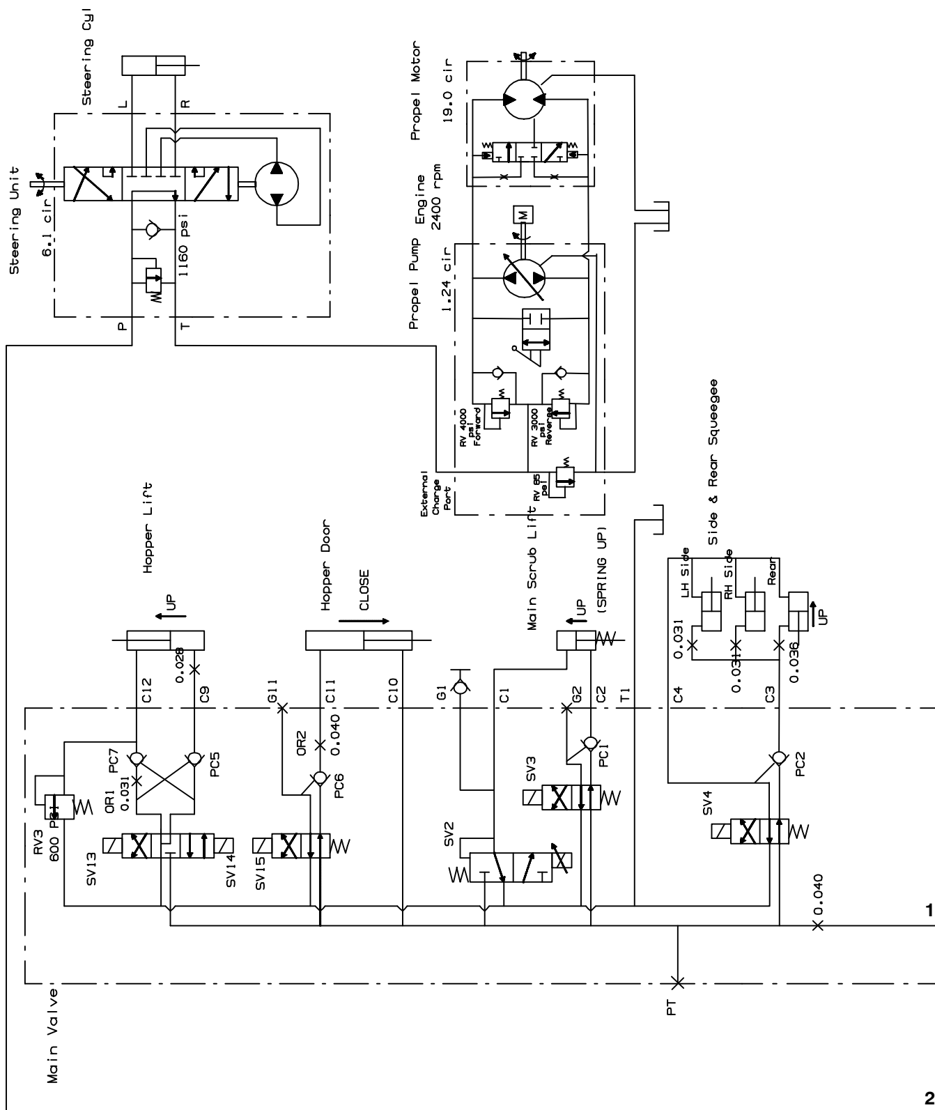
Fig. 74 – Hydraulic Schematic (002700-003297)
